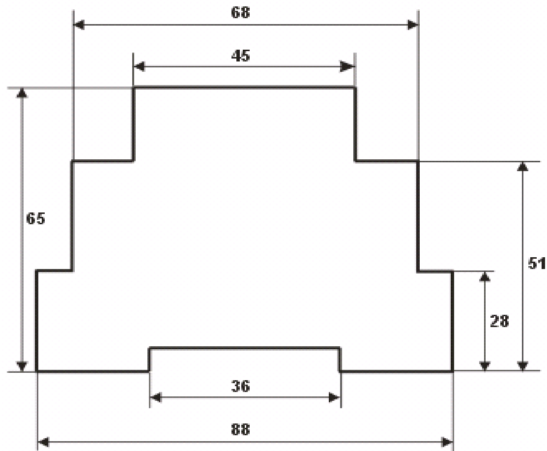
Рисунок 4.1 – Габаритные размеры БП
